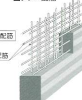
■ダブル配筋
