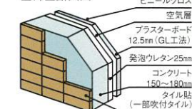
■外壁断面図
