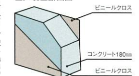
■戸境壁断面図
