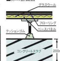
■床の断面図
